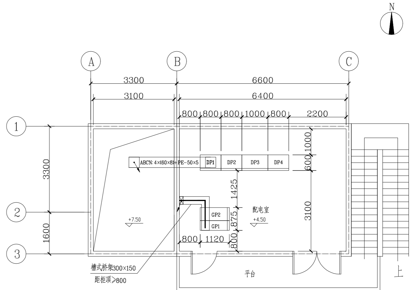
二层设备布置平面图/Scale 1:100
