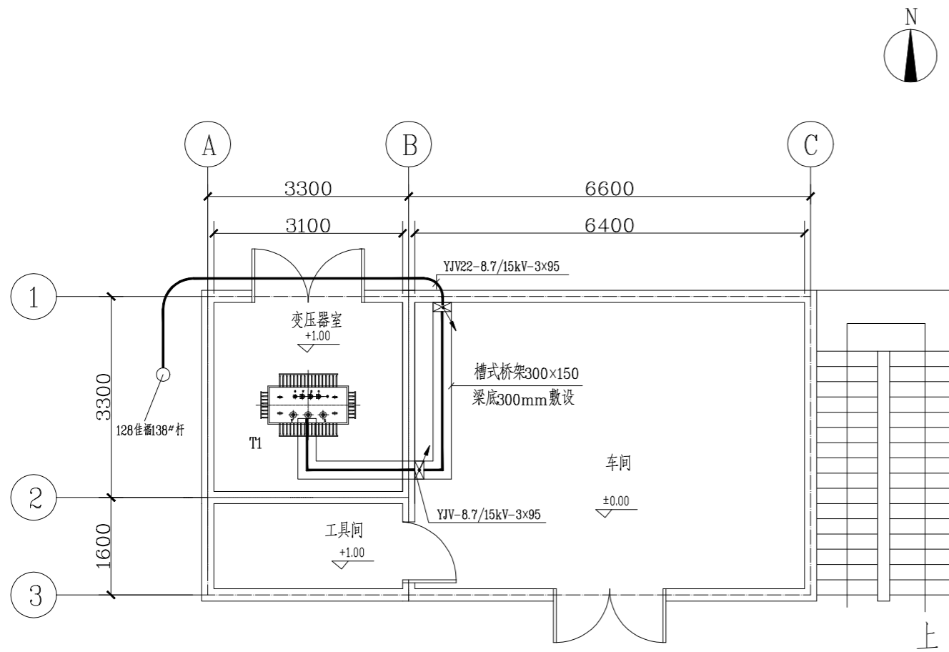
一层设备布置平面图/Scale 1:100
